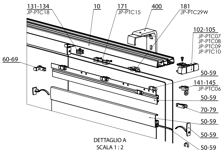
Dettaglio A
