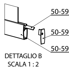
Dettaglio B
